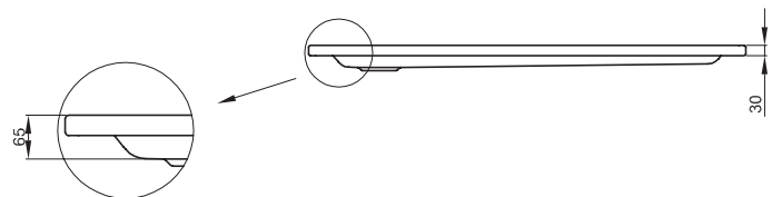
Darstellung ohne Wannenträger
