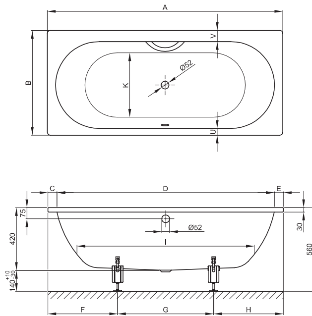
Zeichnung: 157 x 70 cm, Bestell-Nr. 2590
