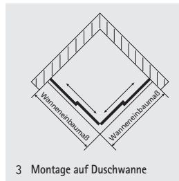
3 Montage auf Duschwanne
