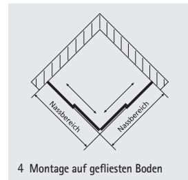
4 Montage auf gefliesten Boden
