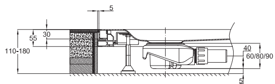
Darstellung mit BETTEINBAUSYSTEM BODENGLEICH
