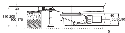
Darstellung mit BETTEFUSS-SYSTEM
