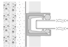
Einbausituation B Montage auf Putz
