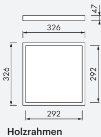
Holzrahmen
