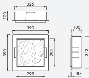
Einbautiefe 10 cm
