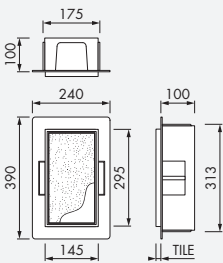
Einbautiefe 10 cm
