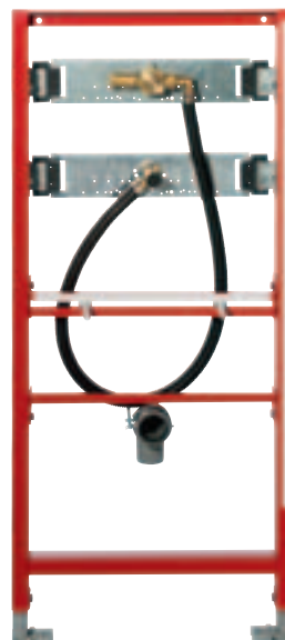
TECEprofil-Urinal-Modul mit TECE-Spülergehäuse Für den Einbau in eine TECEprofil-Vorwand, zur Aufnahme von manuellen und elektronischen Betätigungssystemen. Best.-Nr. 9.320.008
