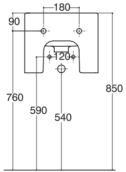
Lavabo cm 37 Washbasin cm 37 Lavabo cm 37 □ cod. 40059 ■ cod. 40060 ■ cod. 40061
