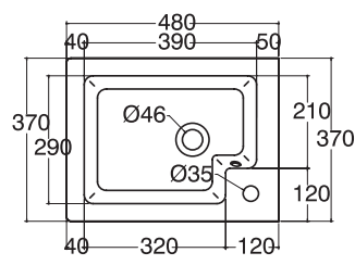
Lavabo cm 37 Washbasin cm 37 Lavabo cm 37 □ cod. 40059 ■ cod. 40060 ■ cod. 40061
