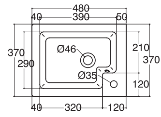
Bidet sospeso Wall hanging bidet Bidet suspendido □ cod. 40059 ■ cod. 40060 ■ cod. 40061
