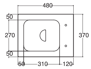
Vaso sospeso Wall hanging w.c. bowl Inodoro suspendido □ cod. 40062 ■ cod. 40063 ■ cod. 40064
