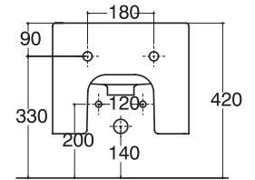
Bidet sospeso Wall hanging bidet Bidet suspendido □ cod. 40059 ■ cod. 40060 ■ cod. 40061
