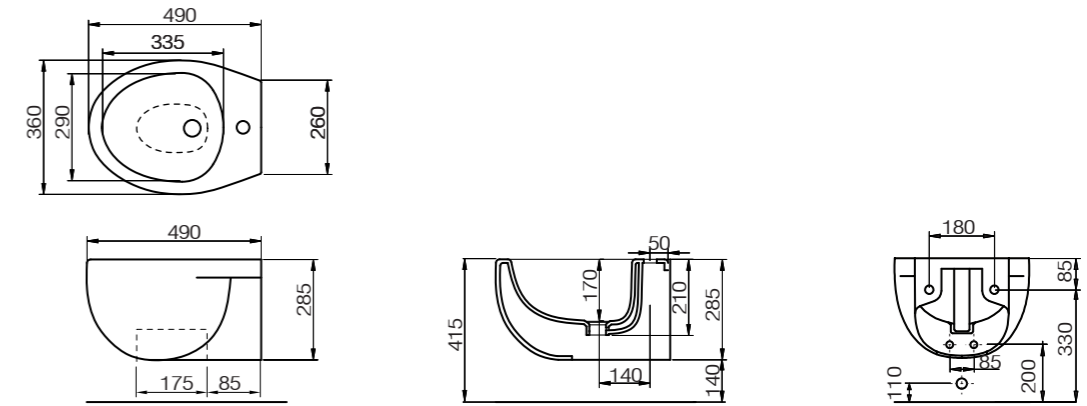
Cento Bidet sospeso Wall hanging bidet Bidé suspendido COD. 40004
