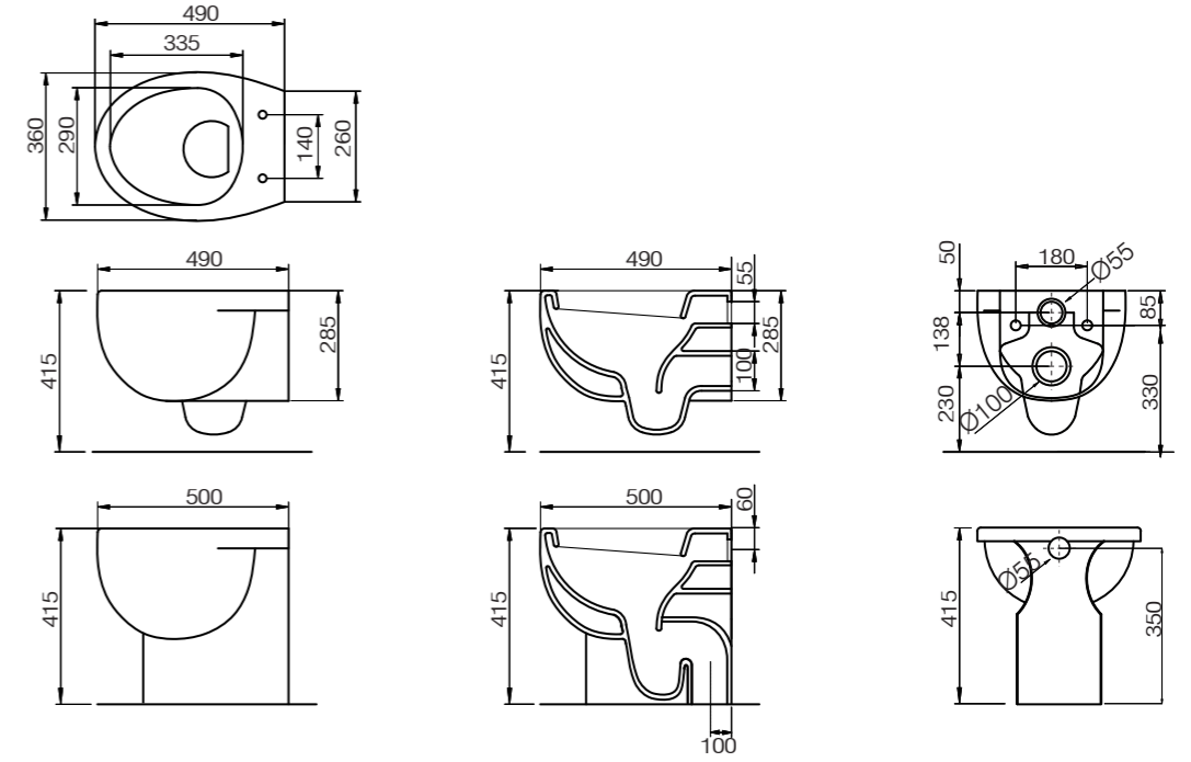
Cento Vaso sospeso Wall hanging w.c. bowl Inodor o suspendido COD. 40002
