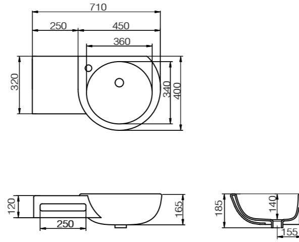
Cento Lavabo SX Washbasin SX Lavabo SX COD. 40006
