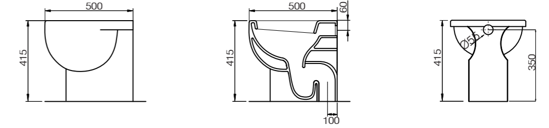
Cento Vaso scarico S W.c. bowl floor trap Inodor o salida V COD. 40000
